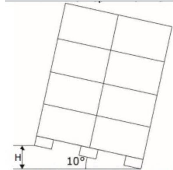
Рис. 47 Грузовая единица в наклонном положении
